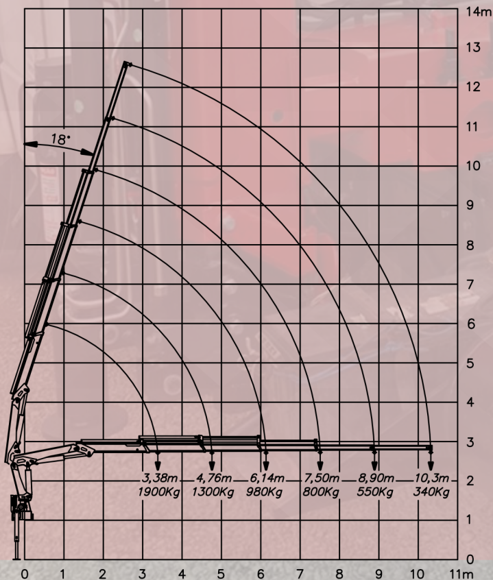
Gráfico de Carga RTmaq 6505
